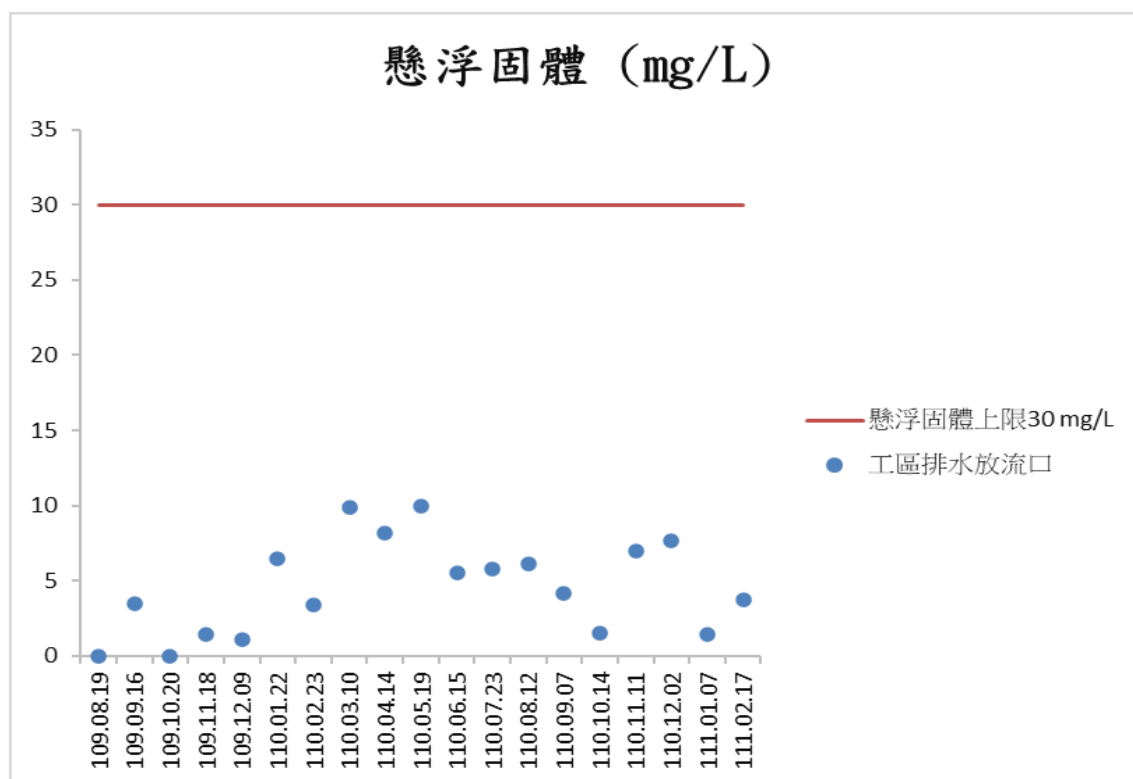
圖 2-9 工區排水放流口監測結果—懸浮固體
