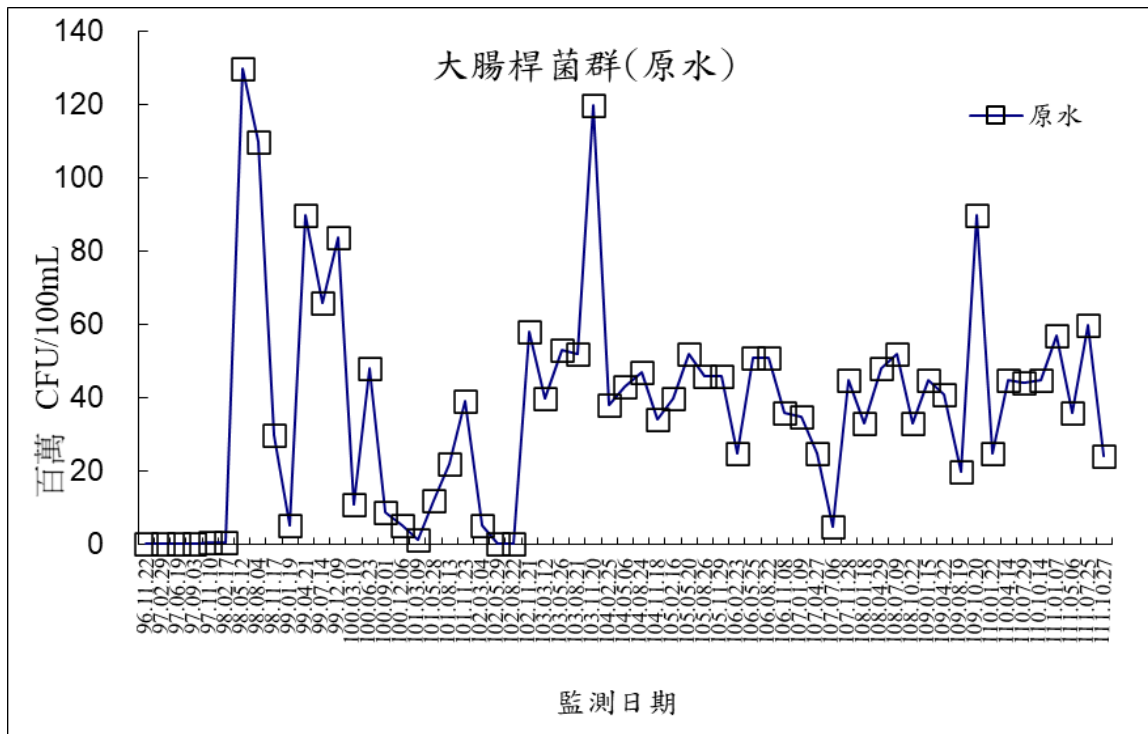
圖 2-5 原水監測結果-大腸桿菌群
