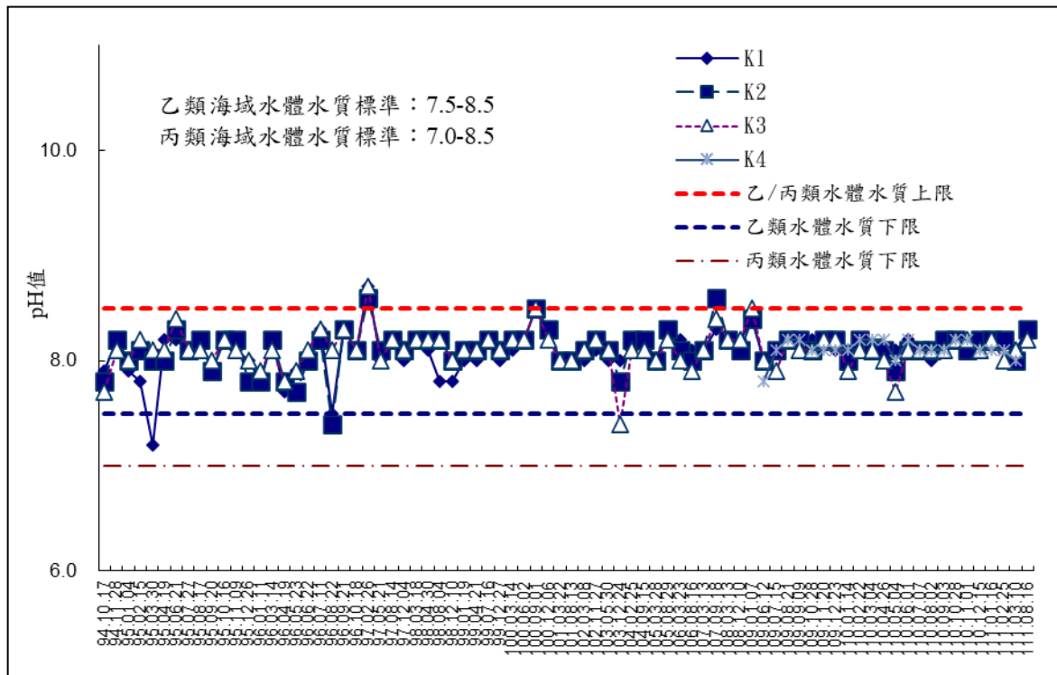
圖 2-14 海域水質監測-pH
