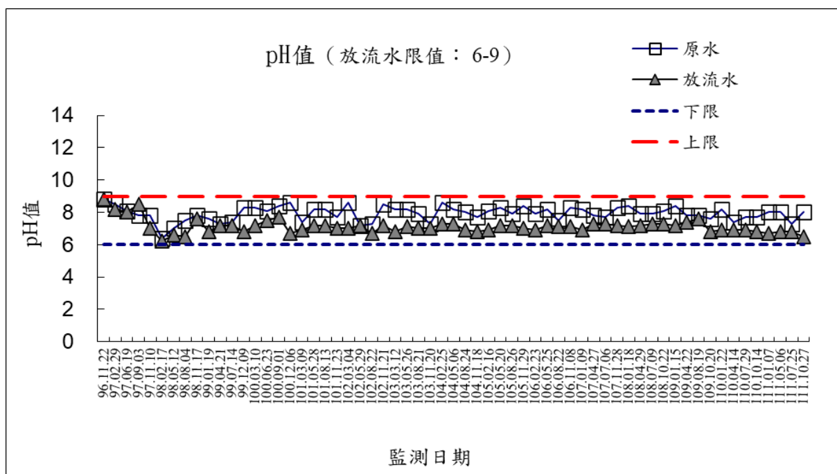
圖 2-1 放流水監測結果-pH
