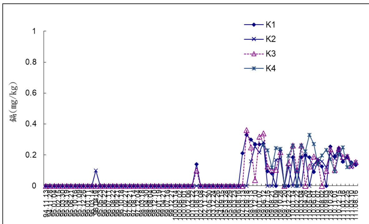
圖 2-29 海域底泥土監測-鉛
