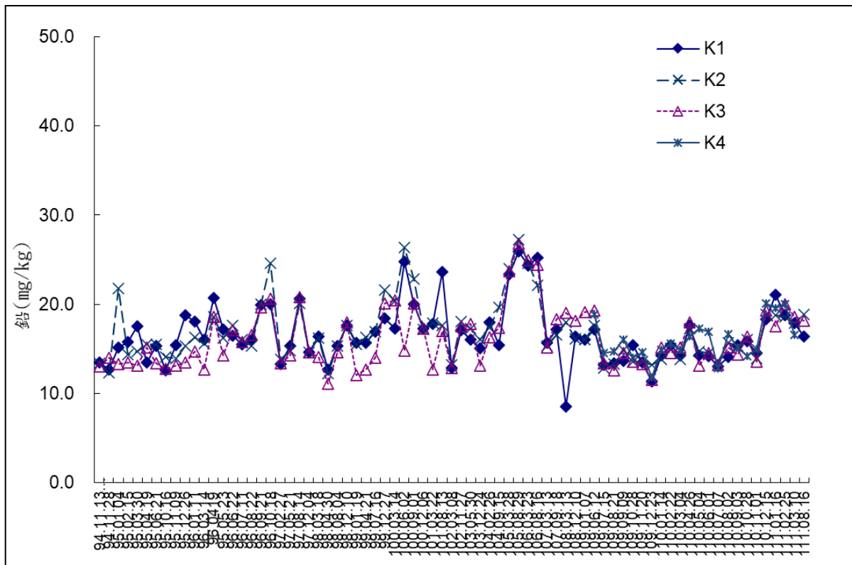
圖 2-27 海域底泥土監測-鉛
