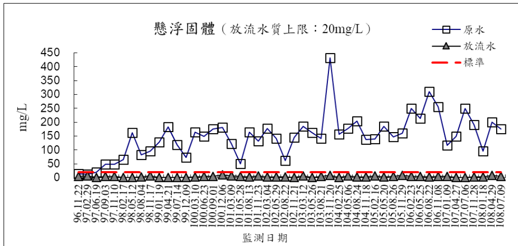
圖 2.3-6 放流水監測結果-懸浮固體
