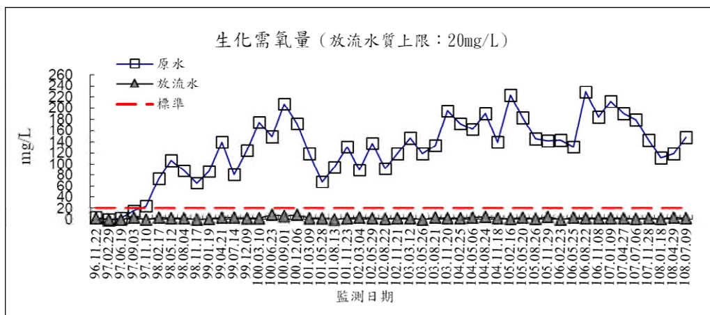
圖 2.3-3 放流水監測結果-生化需氧量
