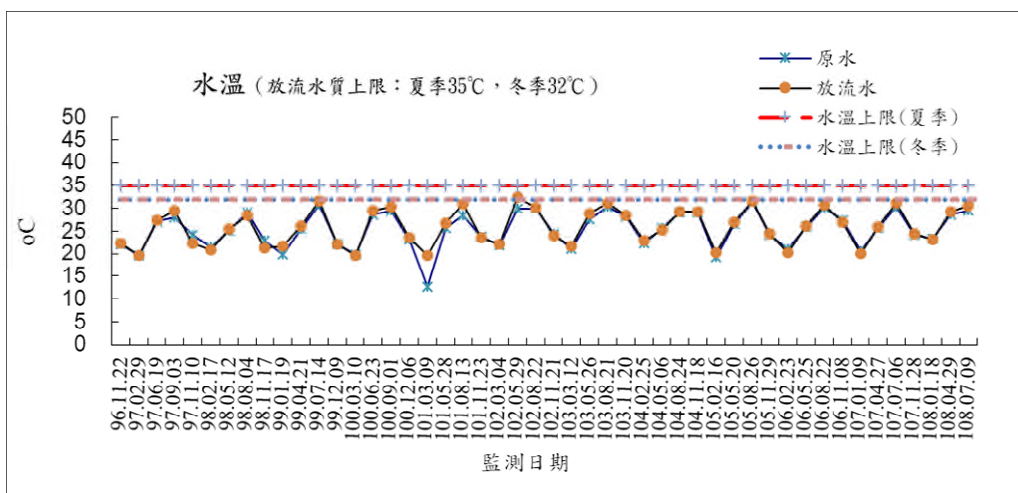
圖 2.3-2 放流水監測結果-水温
