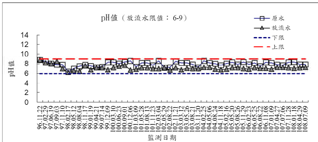
圖 2.3-1 放流水監測結果-pH
