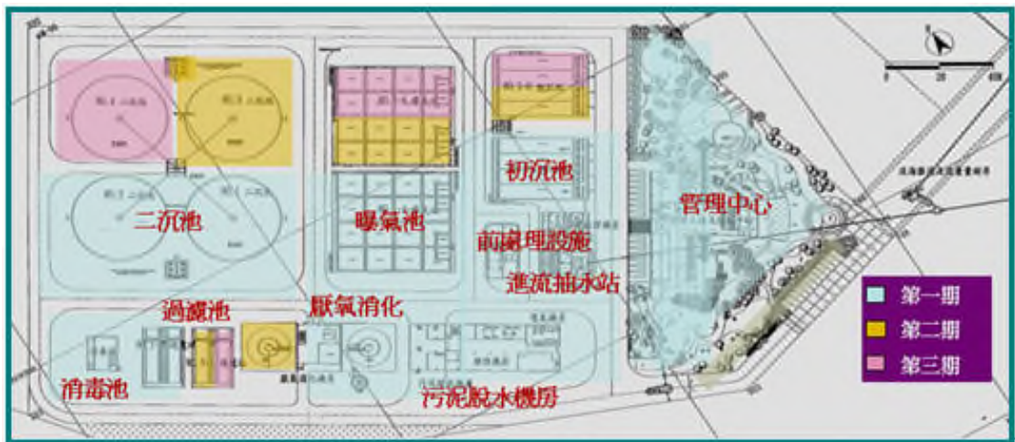
圖 1.1-1 一、二、三期廠區配置圖
