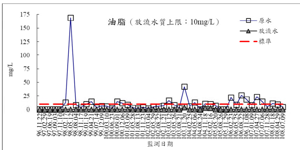
圖 2.3-4 放流水監測結果-油脂
