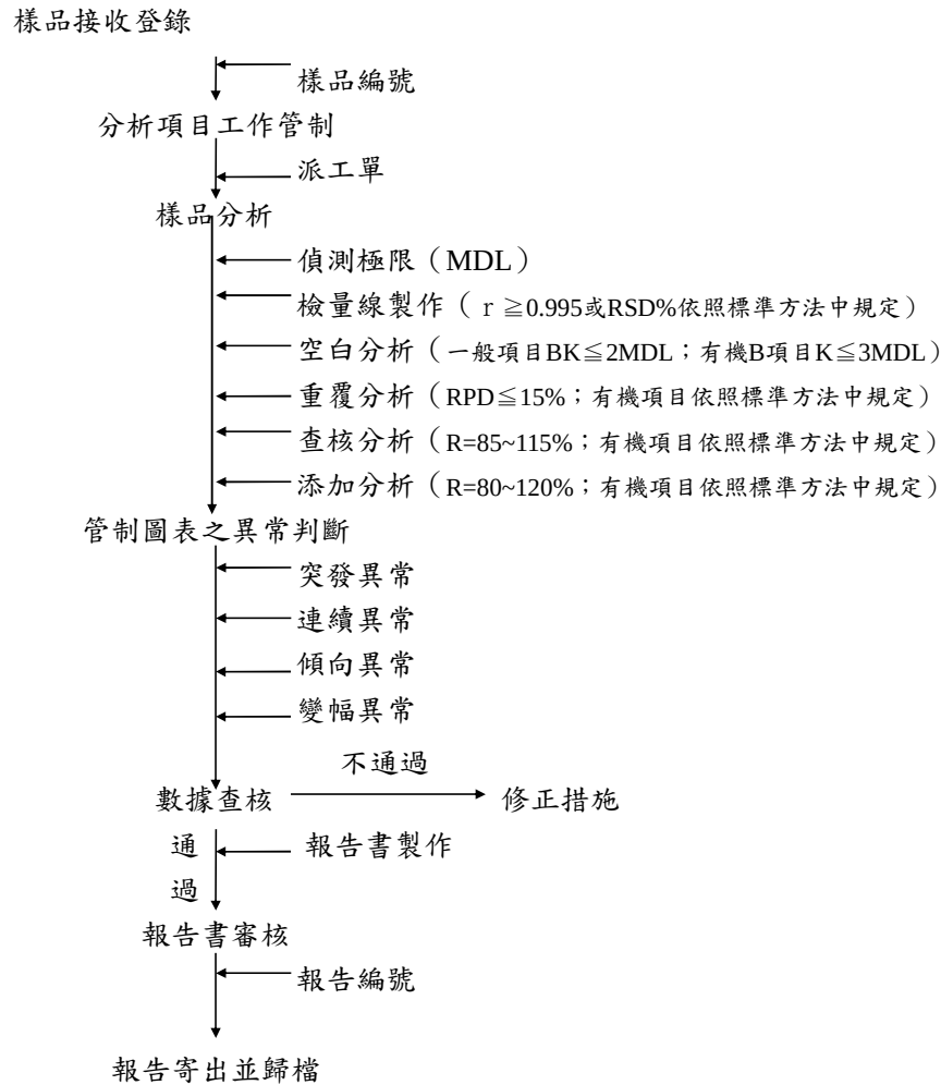
圖 1.5-2 水質之品保/品管作業流程圖
