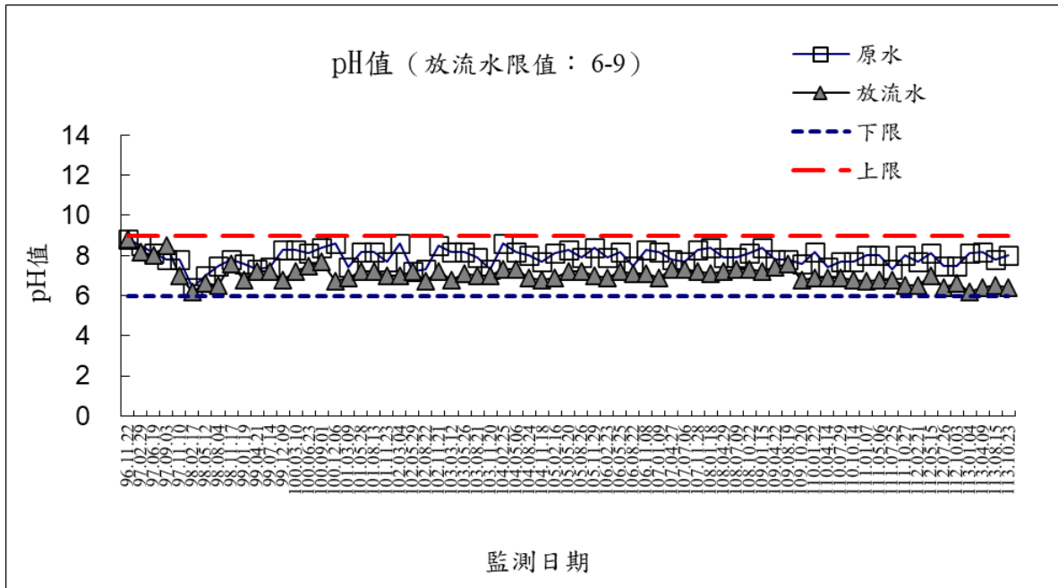
圖 2-1 放流水監測結果-pH
