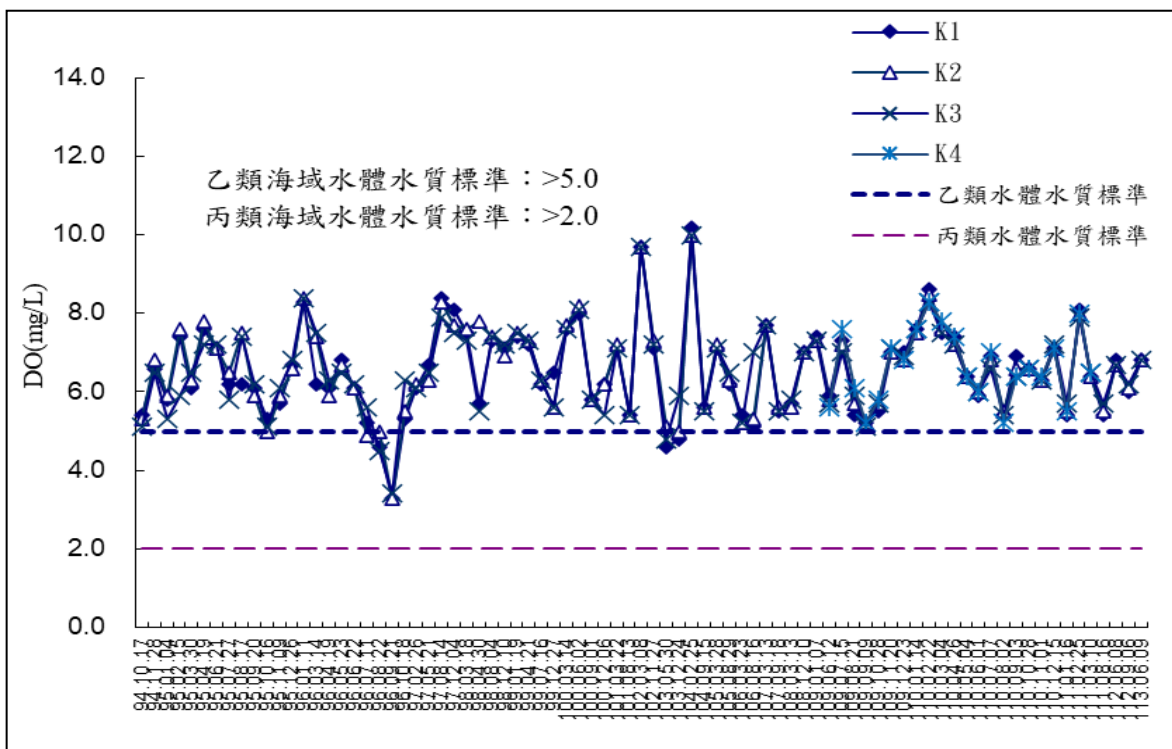
圖 2-15 海域水質監測-溶氧量
