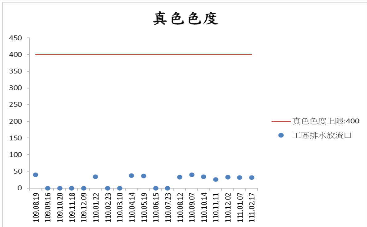
圖 2-11 工區排水放流口監測結果—真色色度
