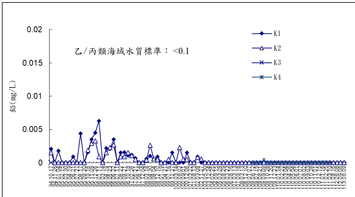
圖 2-21 海域水質監測-鉛
