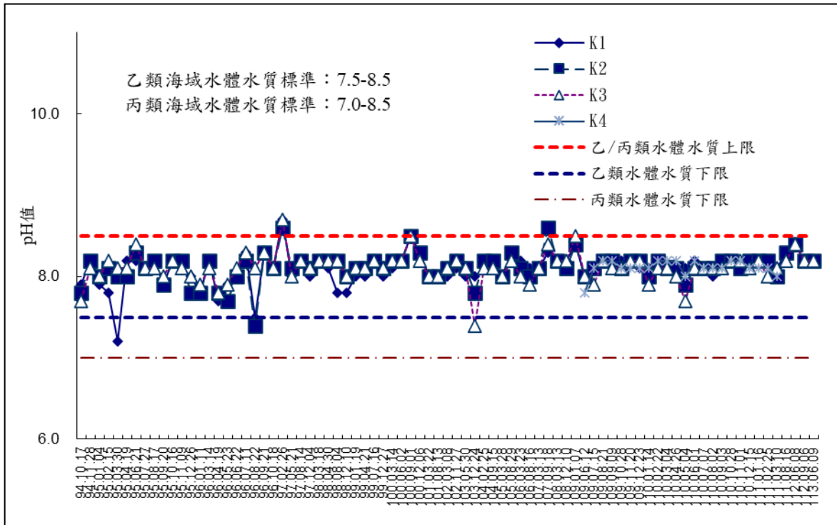
圖 2-14 海域水質監測-pH
