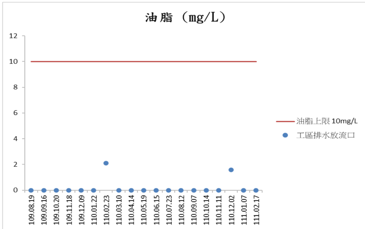
圖 2-10 工區排水放流口監測結果—油脂
