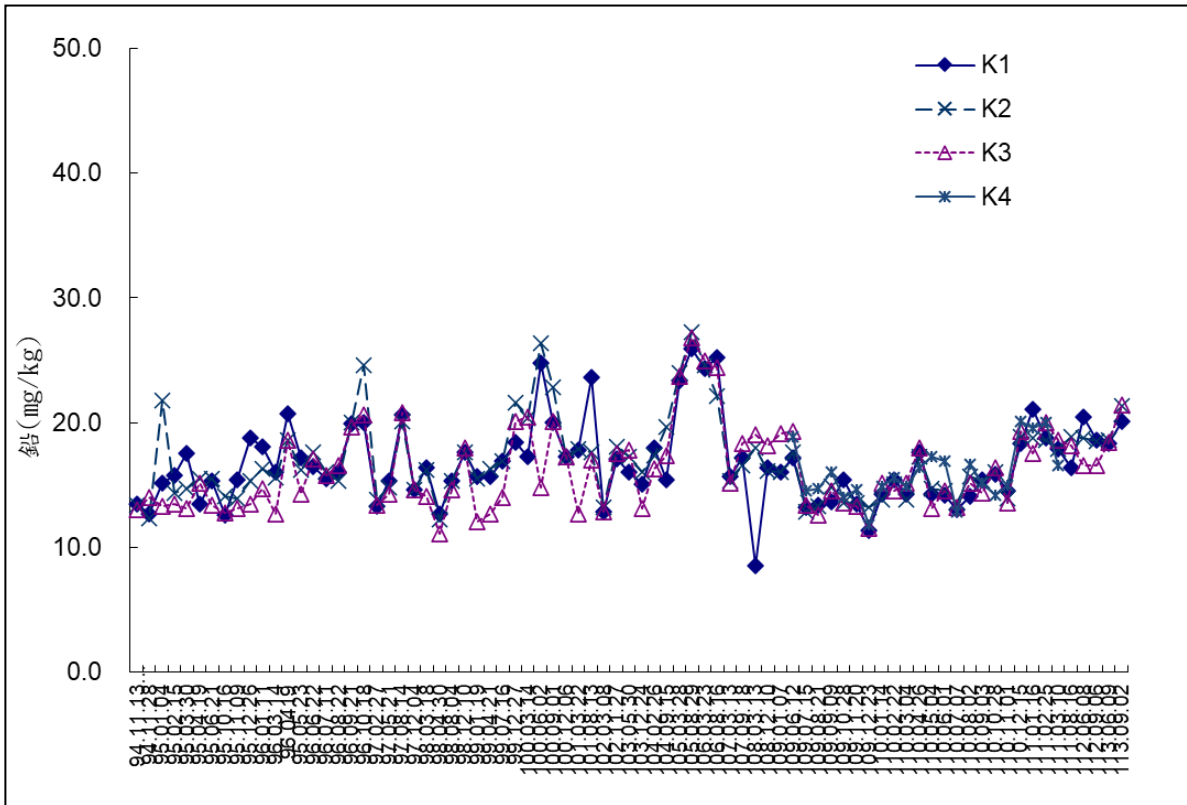
圖 2-27 海域底泥土監測-鉛
