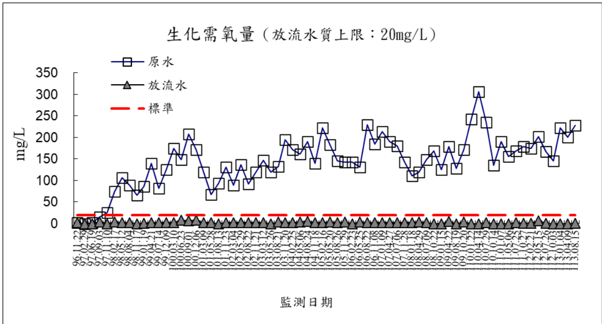
圖 2-3 放流水監測結果-生化需氧量
