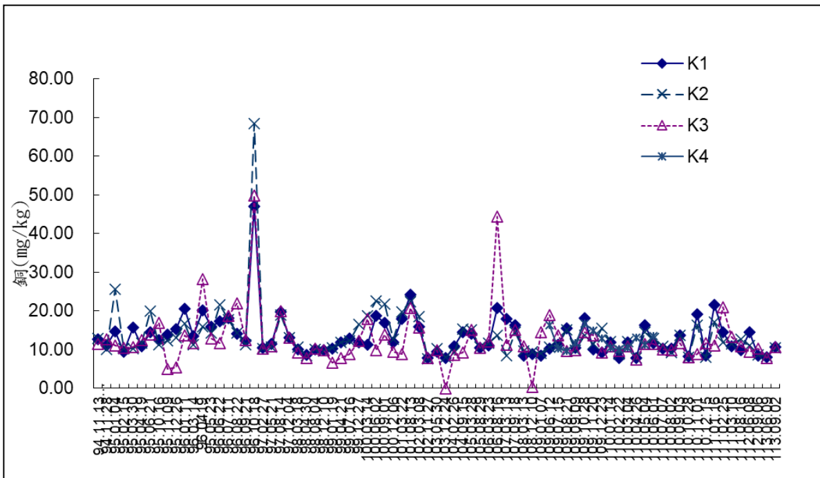
圖 2-28 海域底泥土監測-銅
