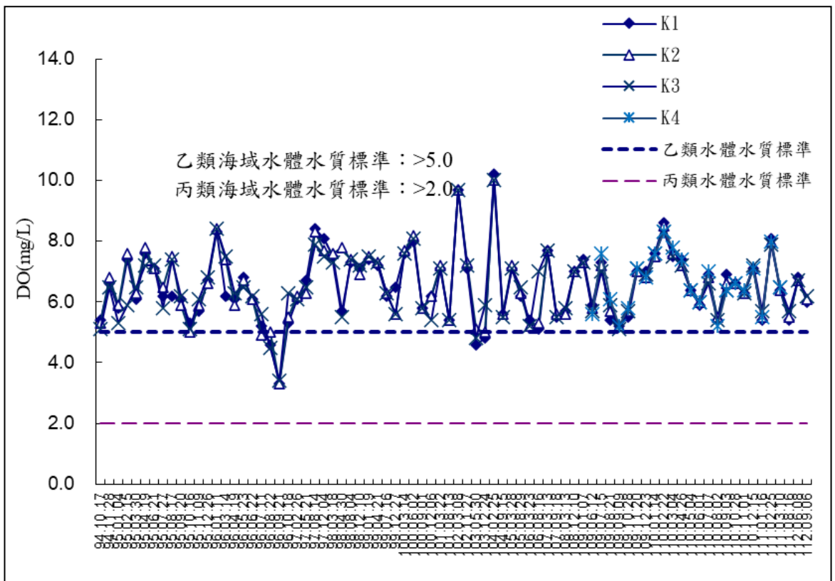
圖 2-15 海域水質監測-溶氧量
