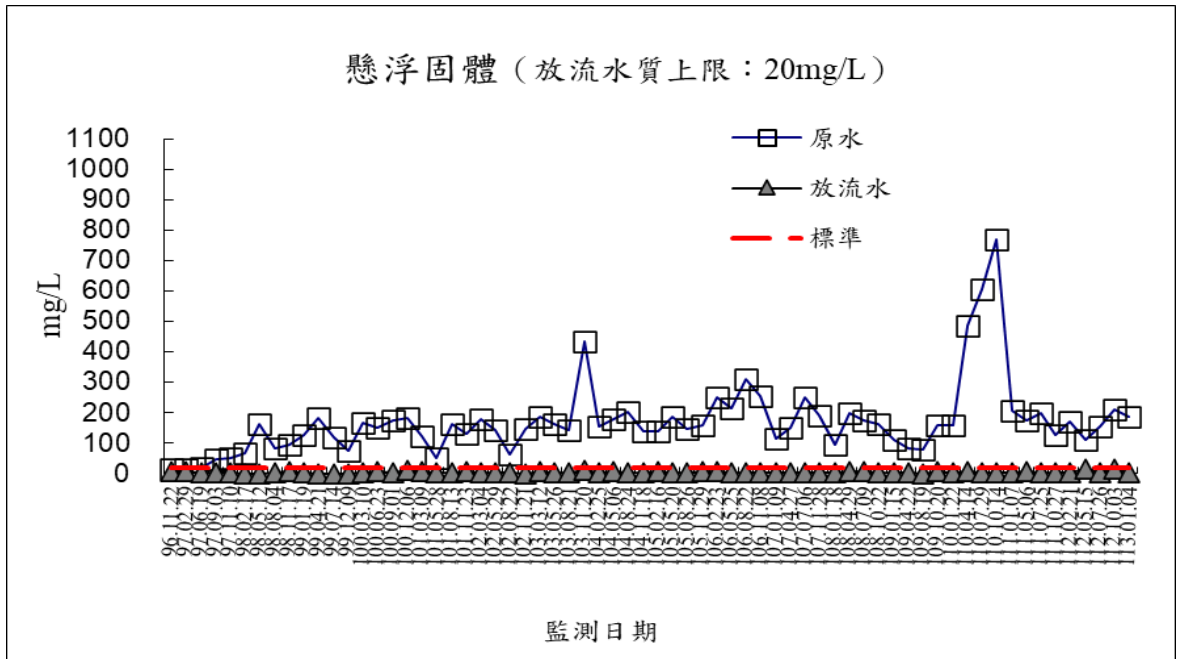
圖 2-7 放流水監測結果-懸浮固體
