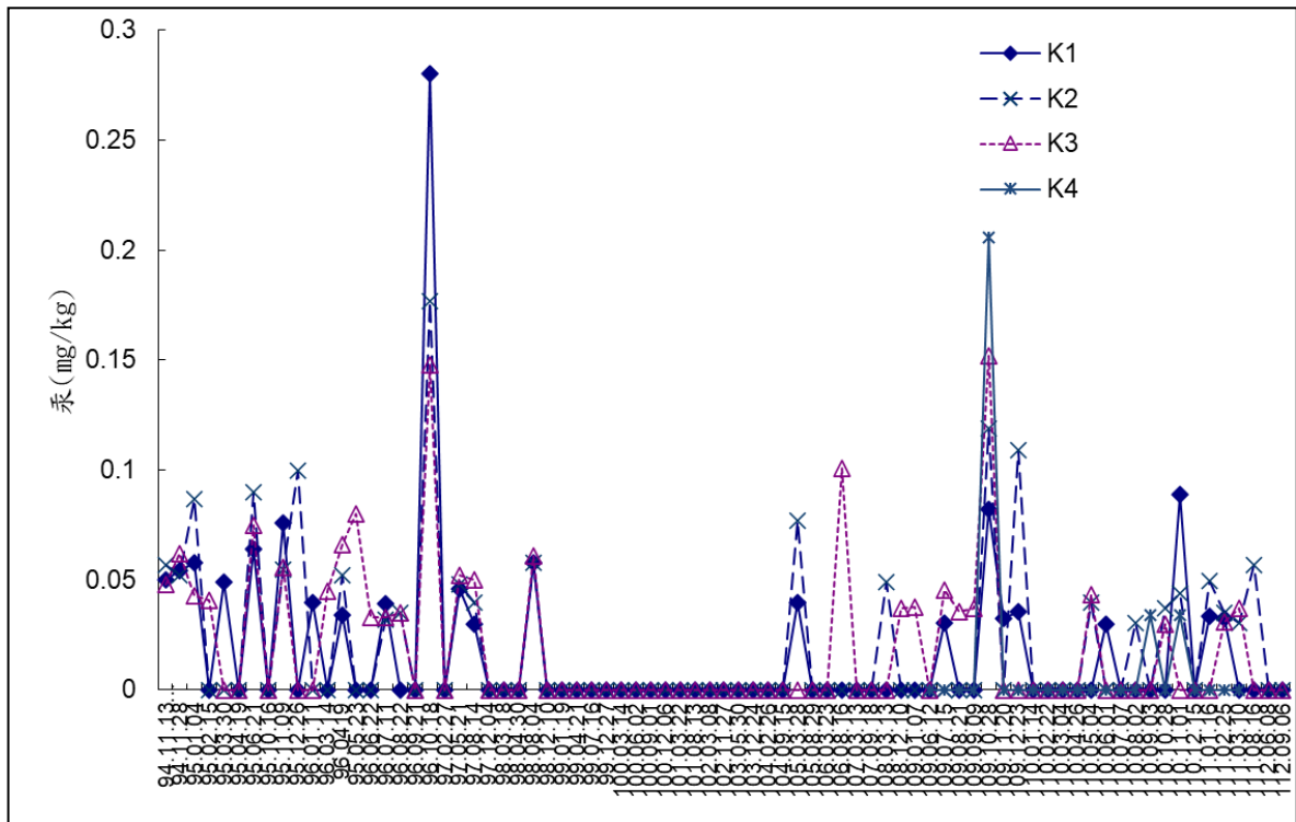
圖 2-25 海域底泥土監測-汞
