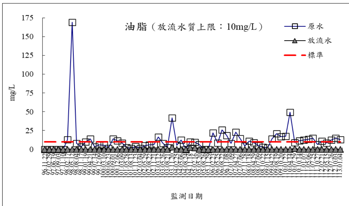
圖 2-4 放流水監測結果-油脂
