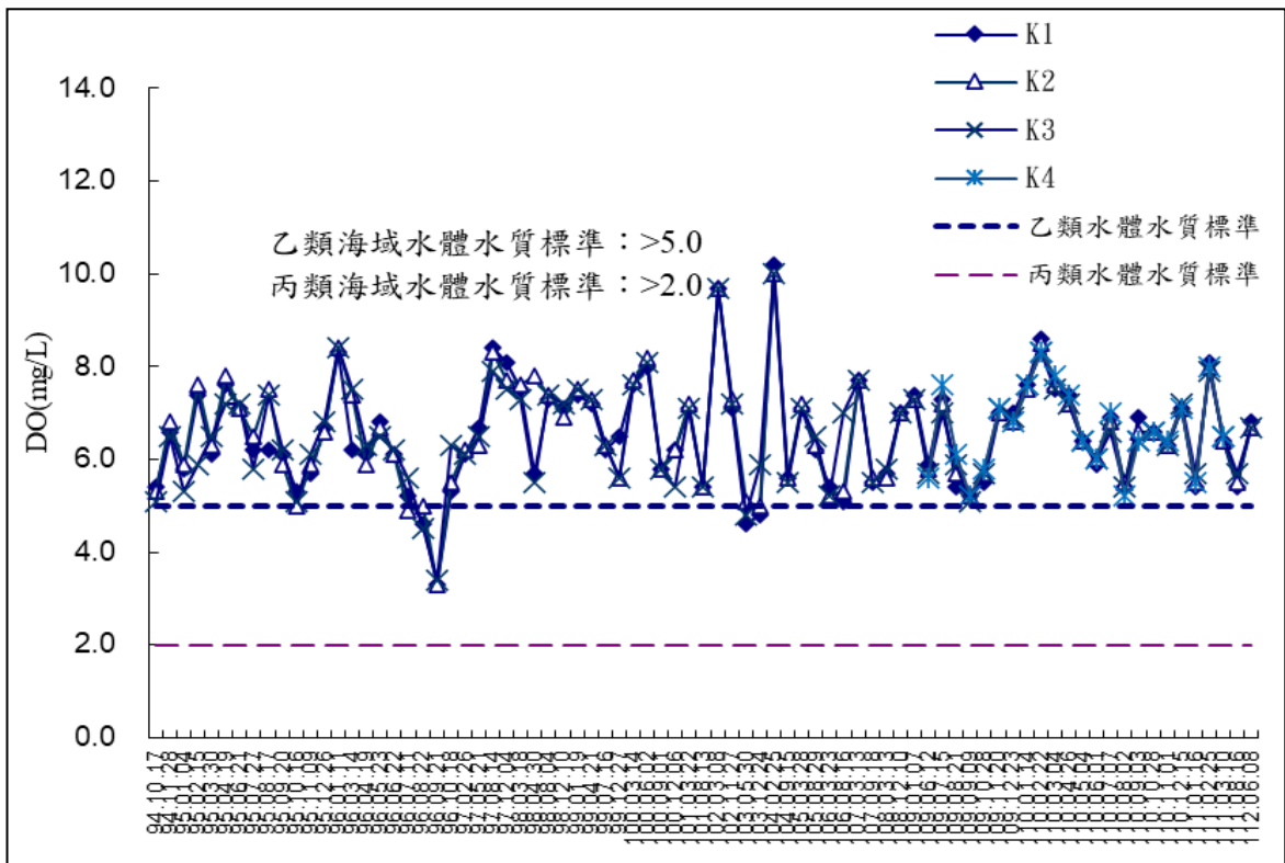
圖 2-15 海域水質監測-溶氧量
