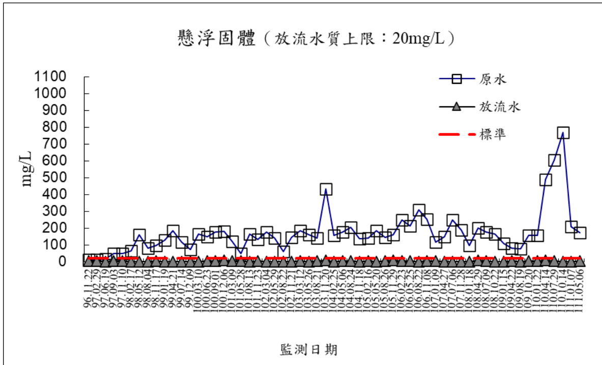
圖 2-7 放流水監測結果-懸浮固體
