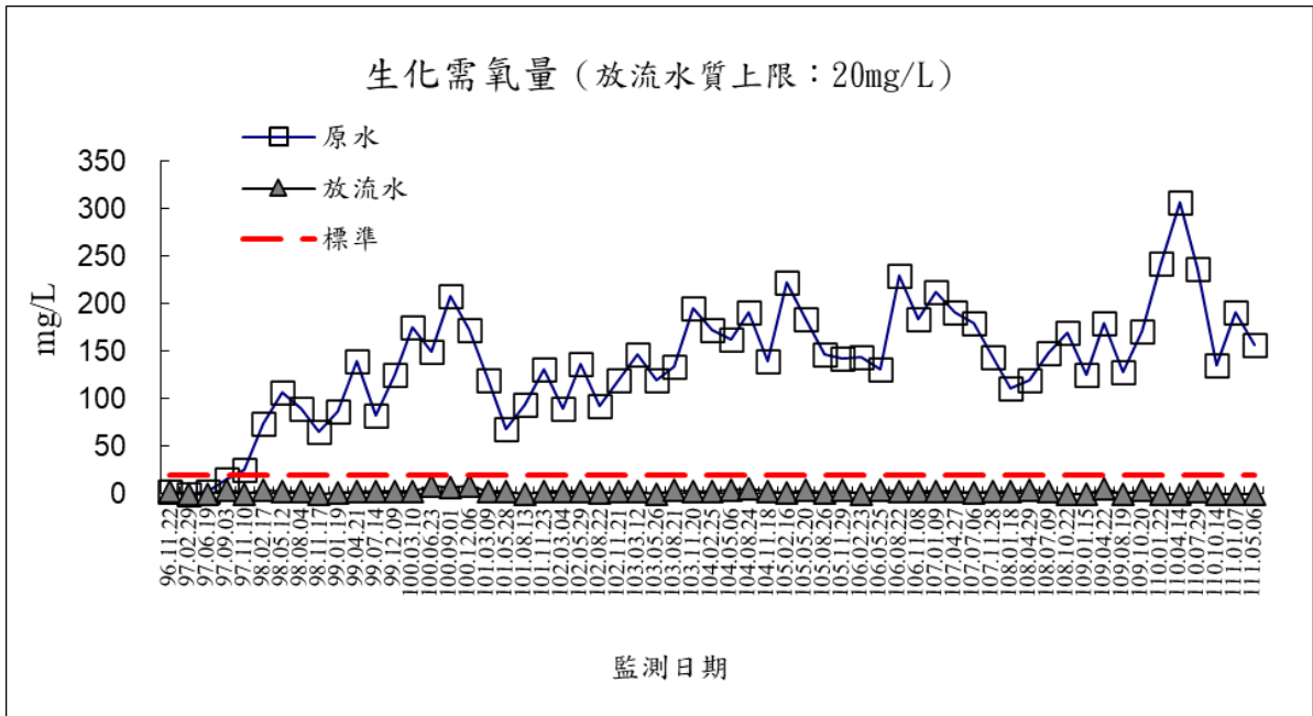
圖 2-3 放流水監測結果-生化需氧量
