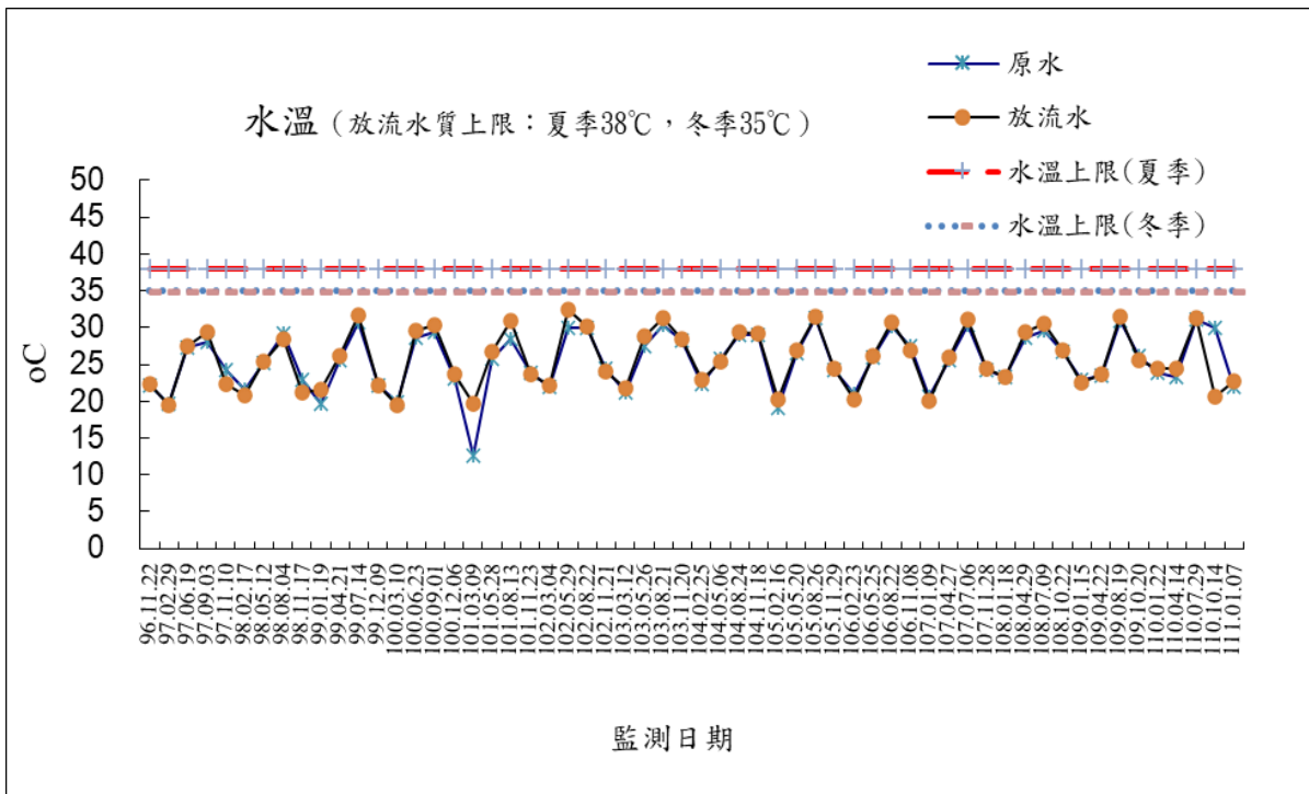
圖 2-2 放流水監測結果-水溫
