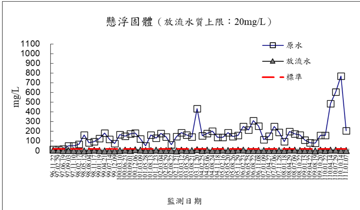
圖 2-7 放流水監測結果-懸浮固體
