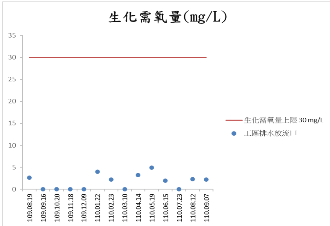
圖 2-12 工區排水放流口監測結果—生化需氧量
