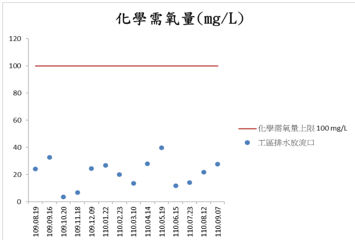
圖 2-13 工區排水放流口監測結果—化學需氧量
