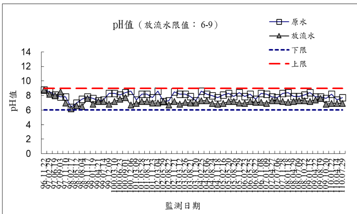
圖 2-1 放流水監測結果-pH
