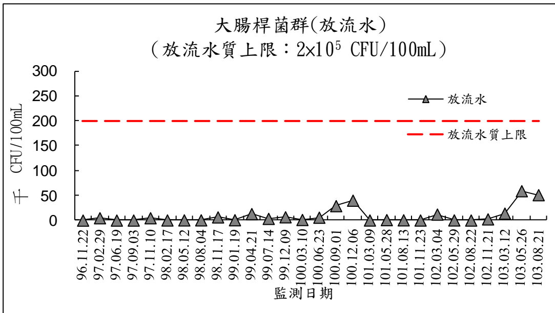
圖 2.3-5 放流水監測結果-大腸桿菌群
