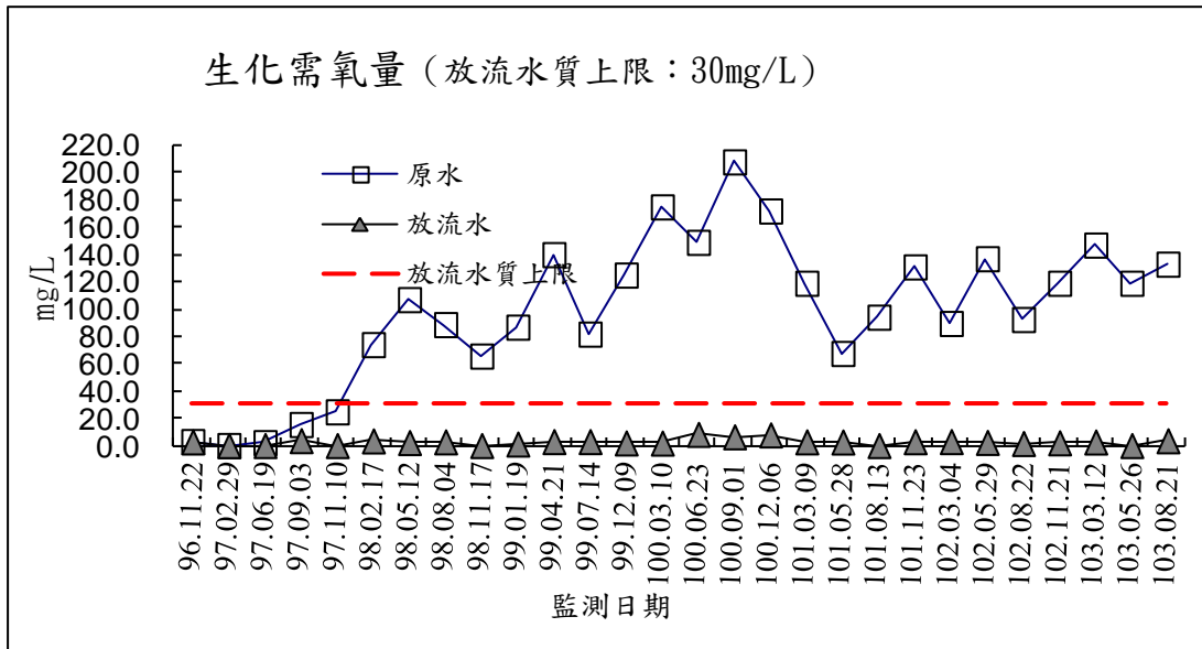
圖 2.3-3 放流水監測結果-生化需氧量
