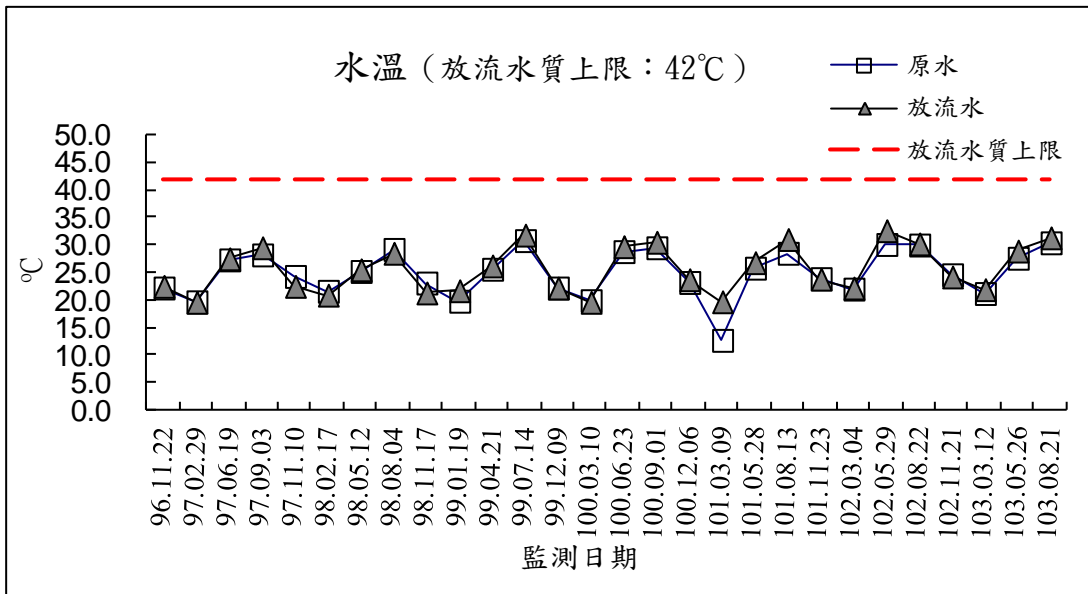
圖 2.3-2 放流水監測結果-水溫
