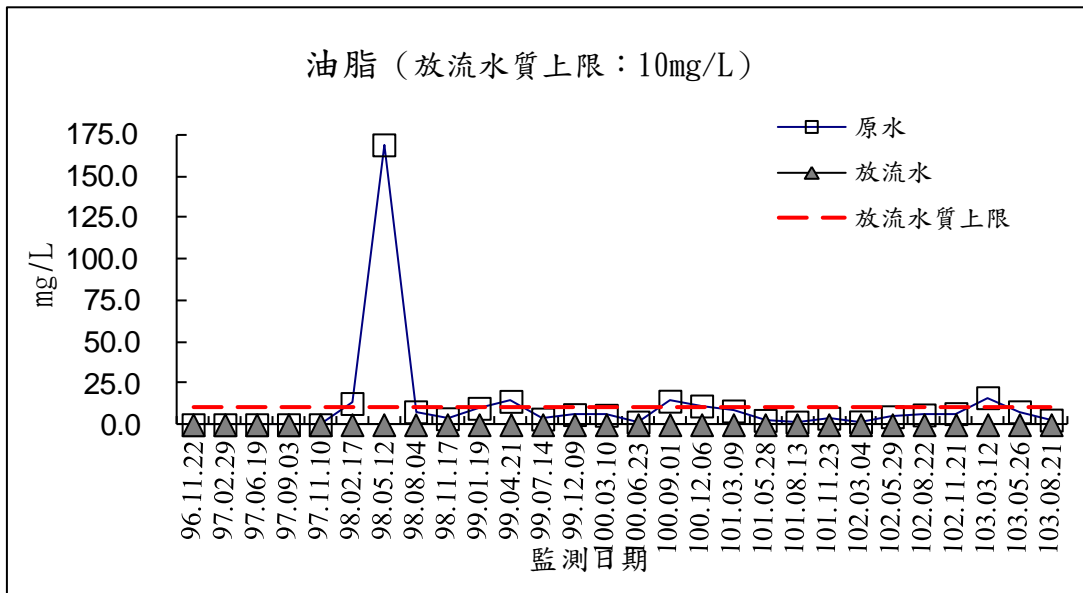
圖 2.3-4 放流水監測結果-油脂
