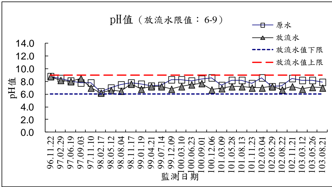
圖 2.3-1 放流水監測結果-pH
